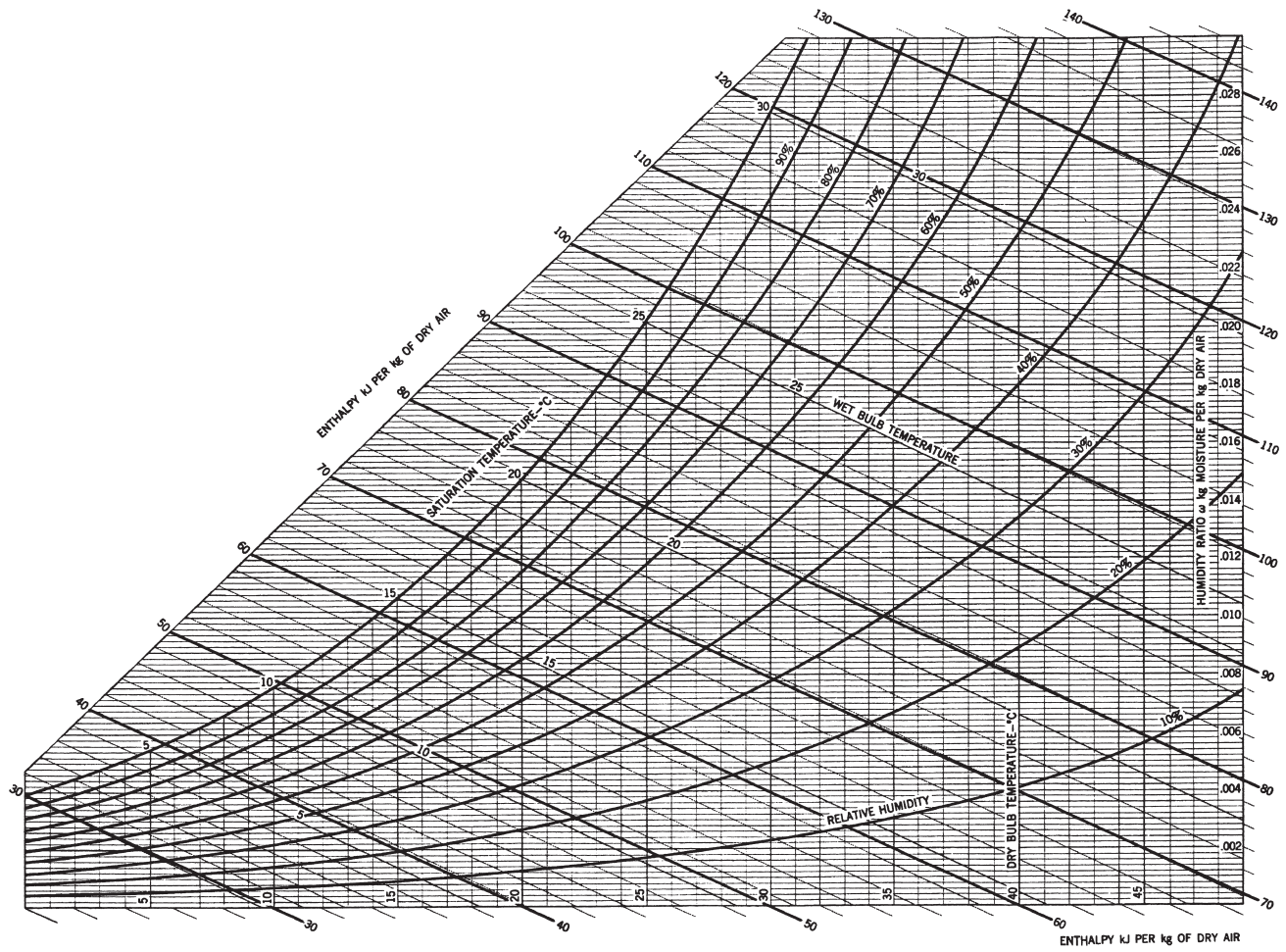
Figura E.4 Carta psicrométrica.
