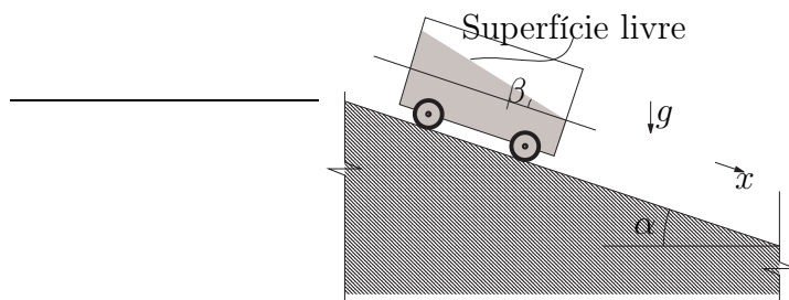
Figura 4.26: Carro com água descendo a ladeira.
