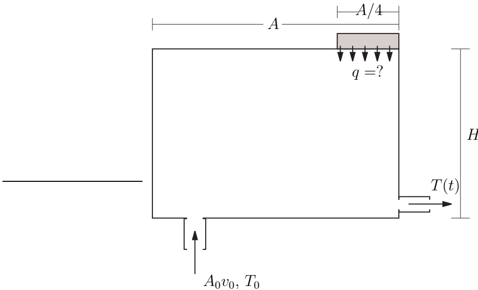
Figura 7.17: Aquecimento de ar circulando recipiente.
