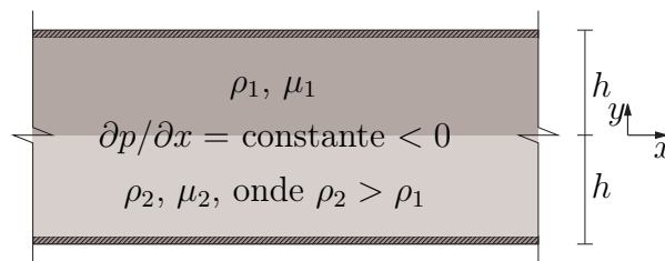
Figura 8.10: Dois fluidos entre placas fixas.
