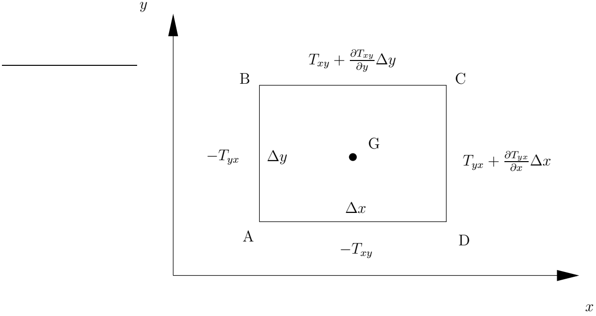
Figura 4.5: Elemento de um fluido. Simetria de \mathbf{T} : T_{xy} = T_{yx} .
