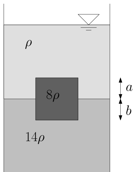
Figura 4.27: bloco flutuante.
