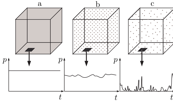
Figura 1.1: Limite de validade da hipótese do contínuo numa câmara com um gás progressivamente evacuado.
