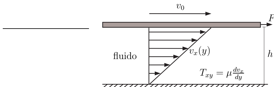
Figura 6.1: O experimento de Newton de transferência de quantidade de movimento.
