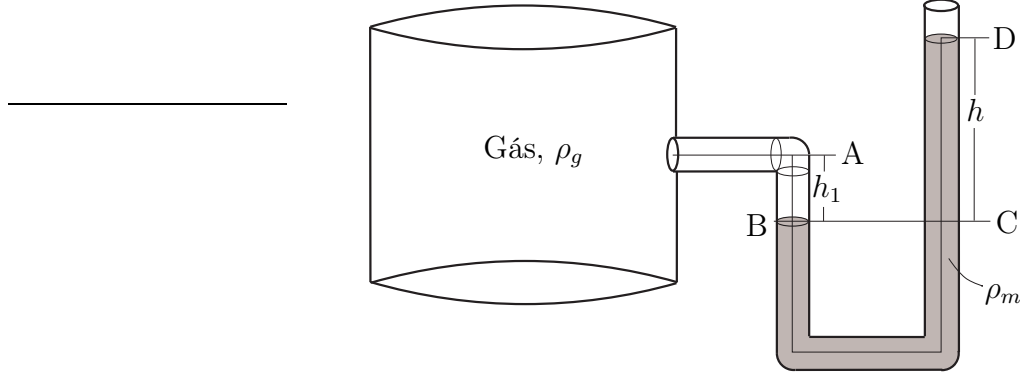
Figura 4.8: Medição de pressão hidrostática. Manômetro em tubo U .
