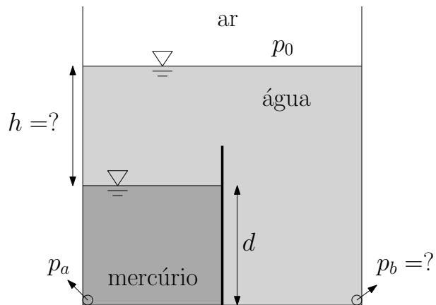
Figura 4.23: Pressão hidrostática.
