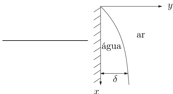
Figura 8.11: Condensação em uma parede.
