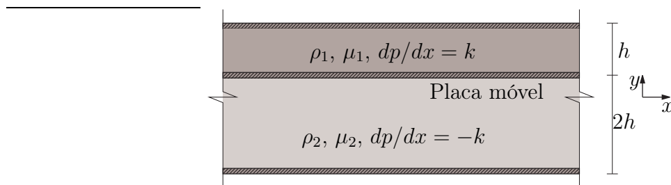
Figura 8.12: Dois fluidos e três placas.
