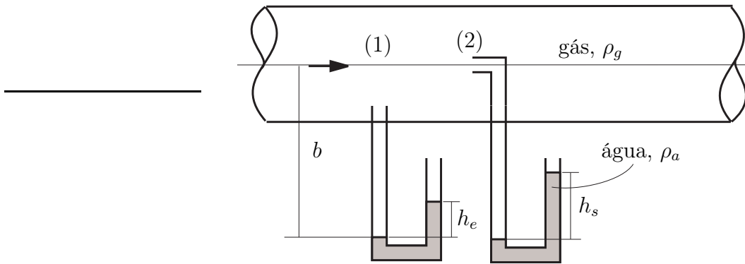
Figura 7.16: Tubo de Pitot.
