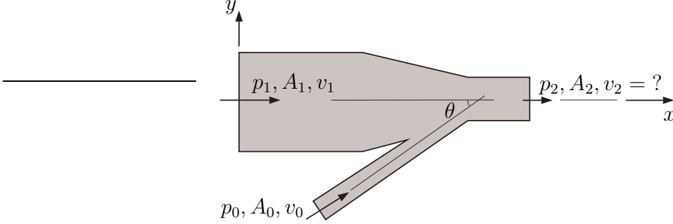
Figura 7.10: Força de um fluido em uma junção.
