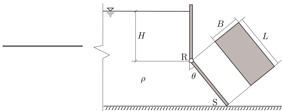
Figura 4.13: Comporta sujeita a pressão hidrostática.
