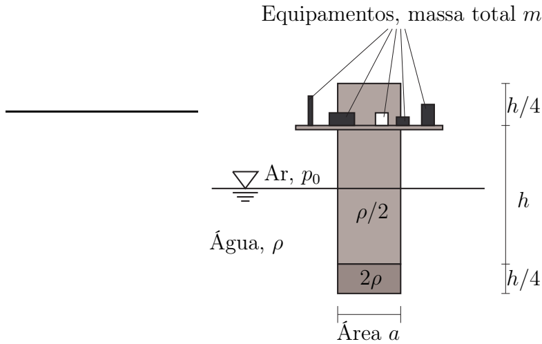
Figura 4.18: Boia suportando equipamentos de medição.
