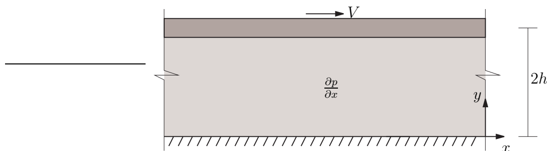
Figura 8.4: Fluido entre placas paralelas sujeito a gradiente de pressão.
