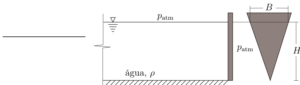
Figura 4.14: Determinação das forças de pressão em uma comporta triangular.
