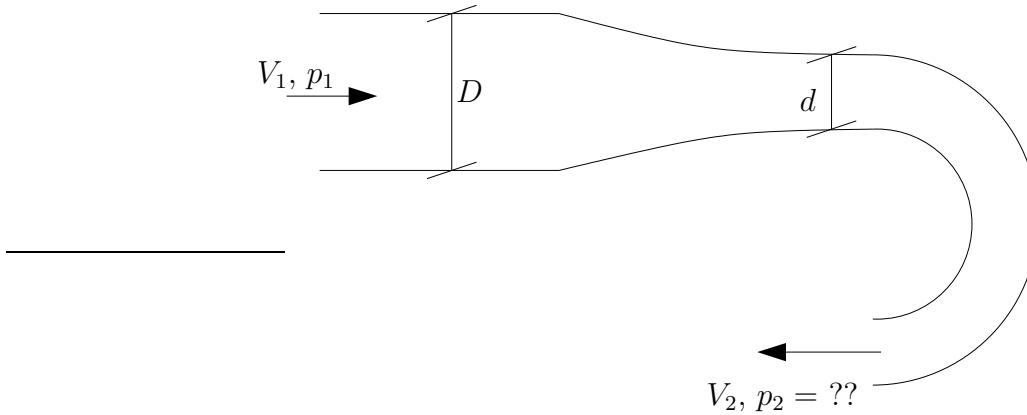
Figura 7.25: Força em um trecho conduto.
