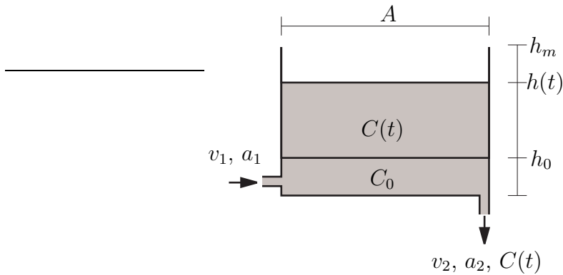
Figura 7.20: Entra água pura – Sai água com cloro.
