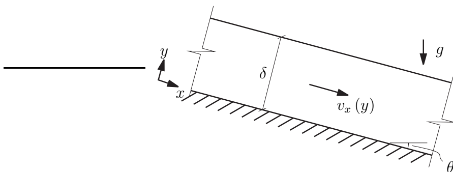
Figura 8.9: Escoamento em plano inclinado.
