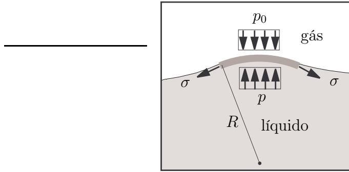
Figura 8.1: Ação da tensão superficial num elemento de uma superfície livre.
