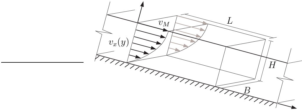
Figura 6.8: Escoamento em um canal com superfície livre.
