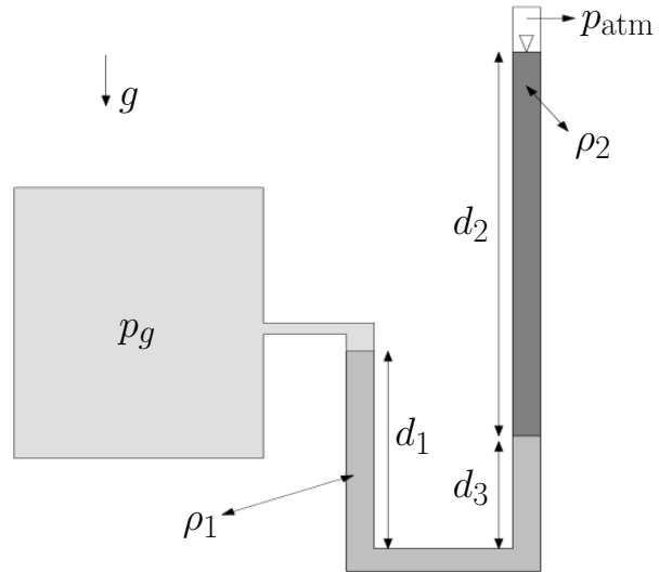
Figura 4.24: Tubo em U.
